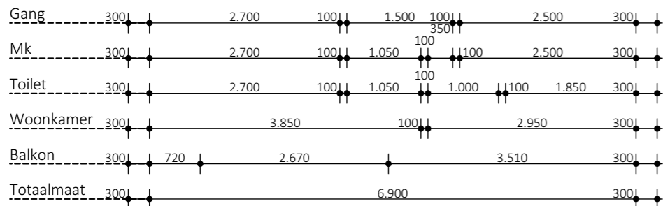
Verdieping tussenwoning type B
