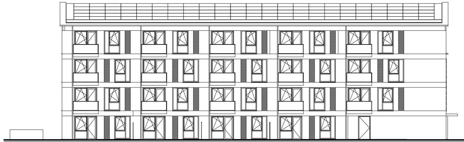
Voorgevel
