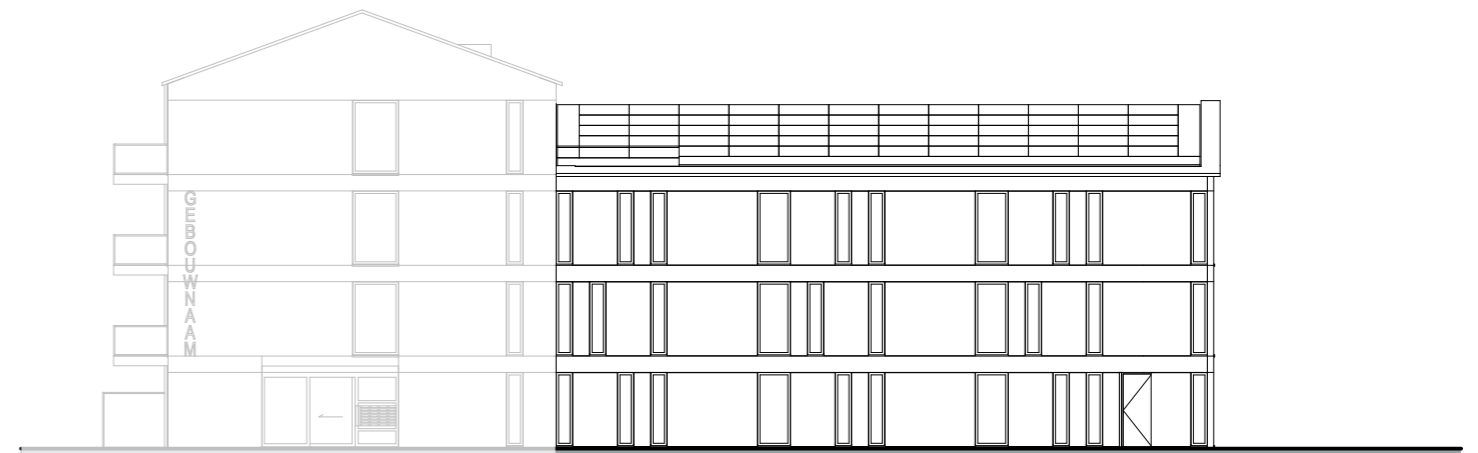
Zijgevel Rechts
