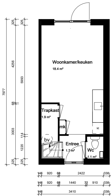
begane grond
