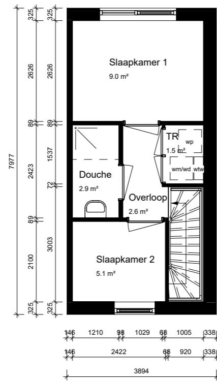
eerste verdieping
