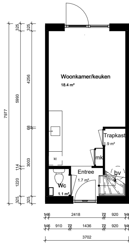
begane grond
