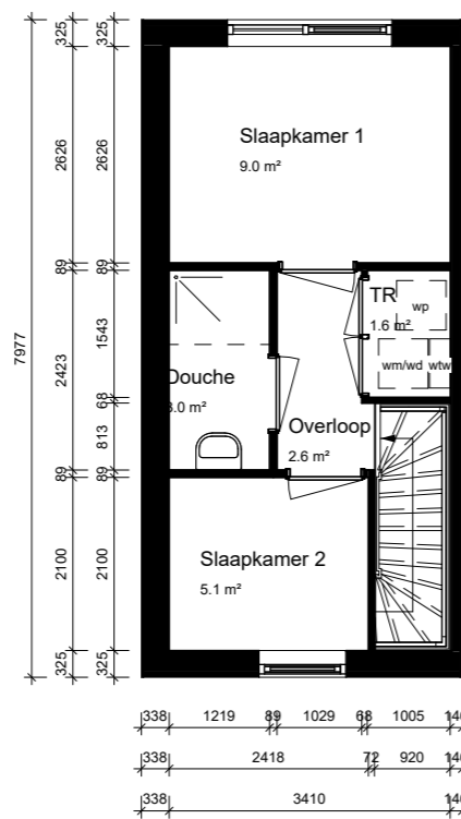
eerste verdieping
