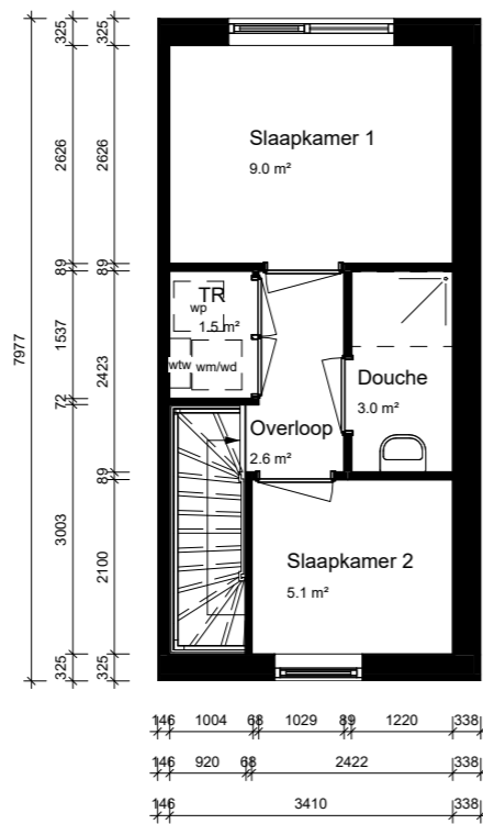
eerste verdieping
