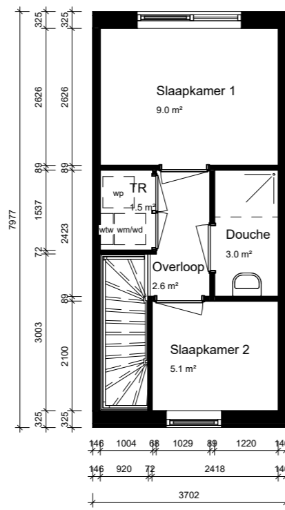
eerste verdieping
