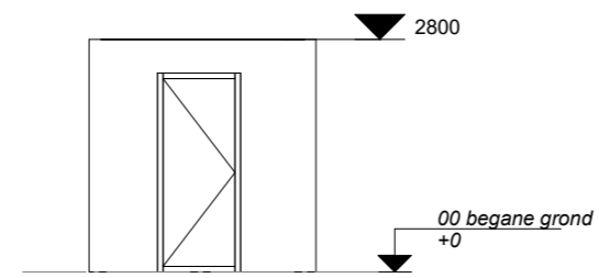
gevel - berging
