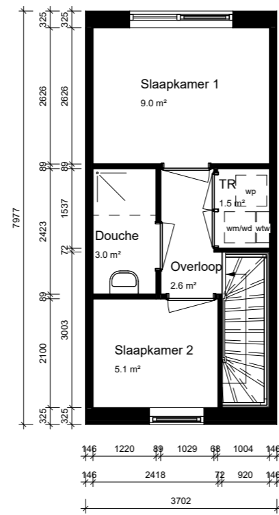
eerste verdieping
