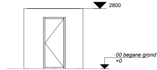
gevel - berging
