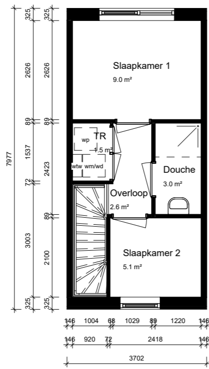
eerste verdieping
