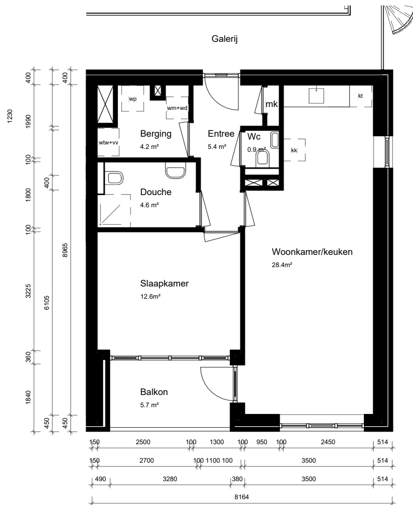
tweede verdieping
