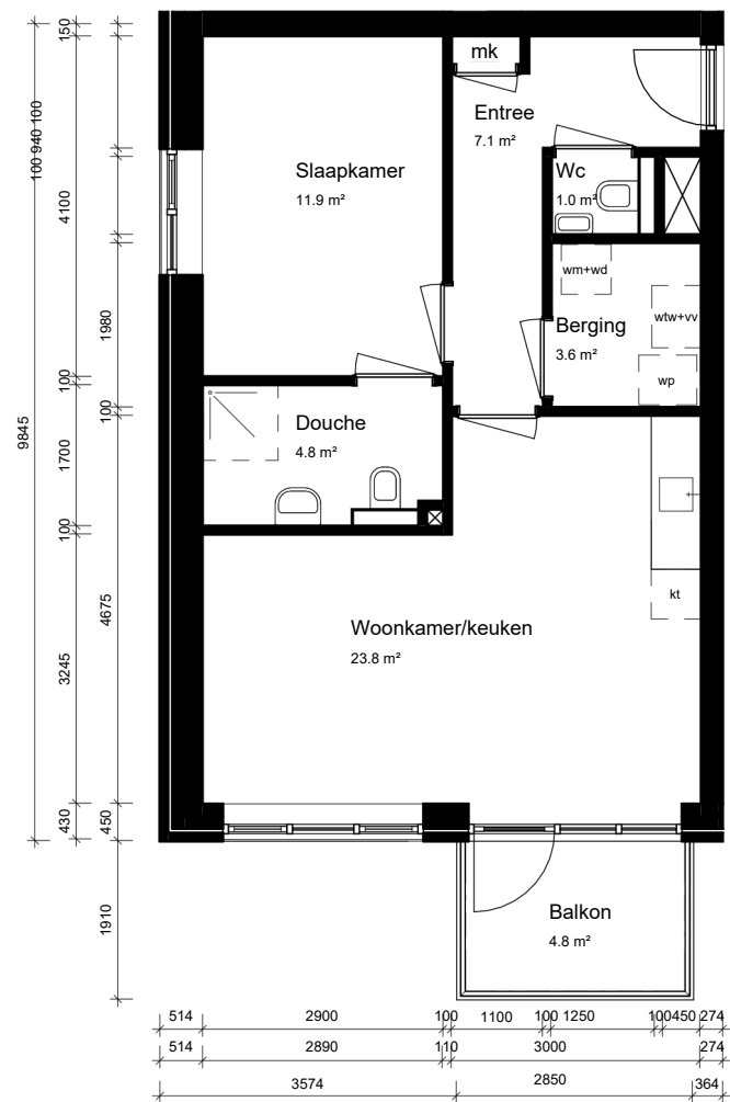
eerste verdieping
