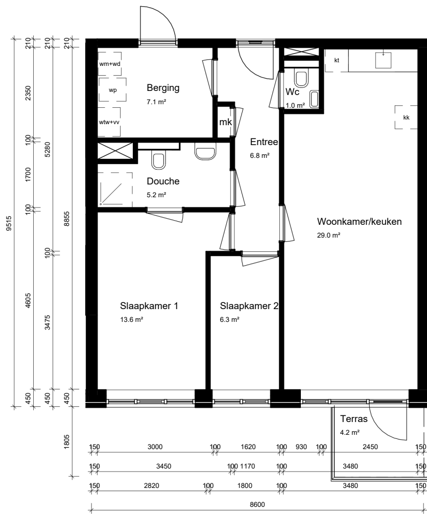
eerste verdieping
