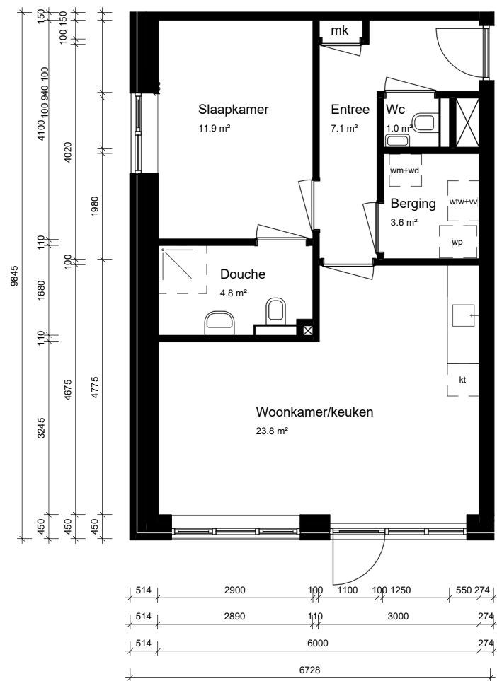
begane grond
