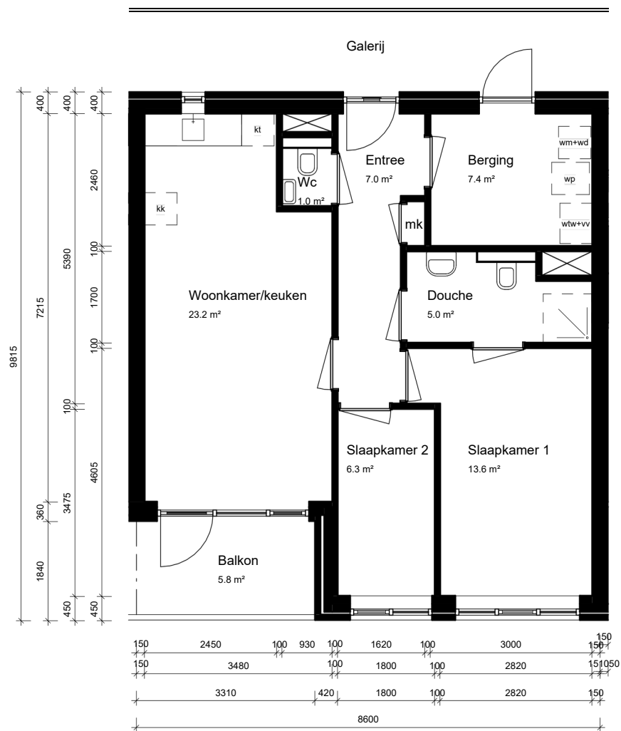
tweede verdieping
