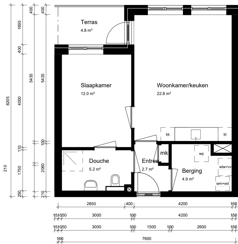
eerste verdieping
