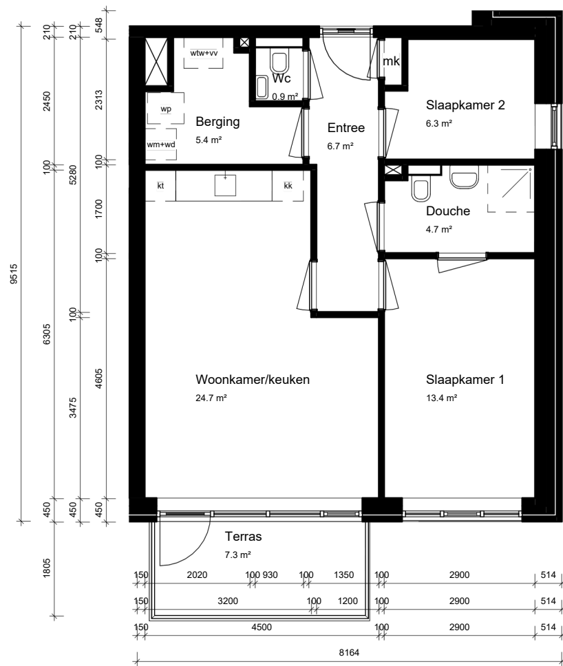
eerste verdieping
