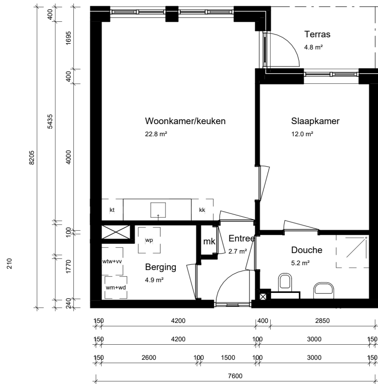
begane grond
