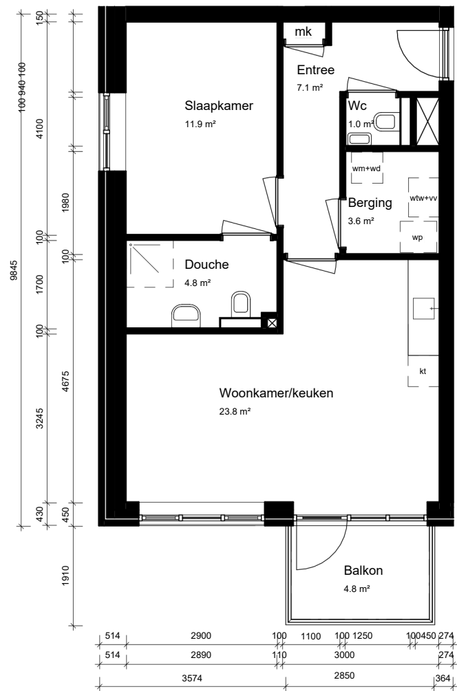
tweede verdieping
