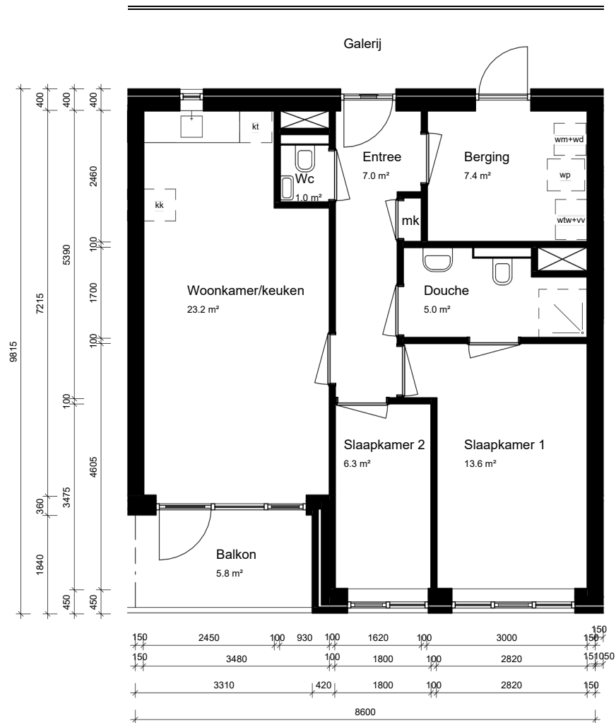
tweede verdieping
