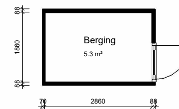
begane grond
