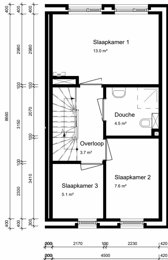
eerste verdieping
