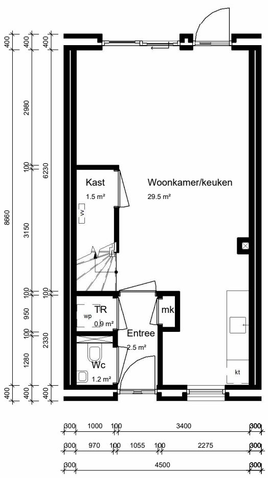
begane grond
