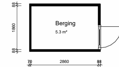
begane grond
