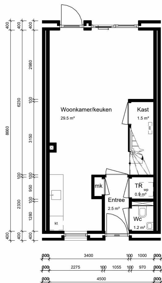
begane grond
