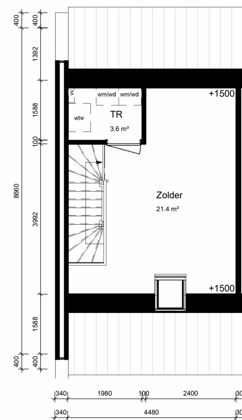
tweede verdieping
