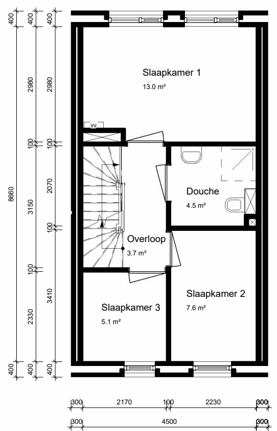
eerste verdieping
