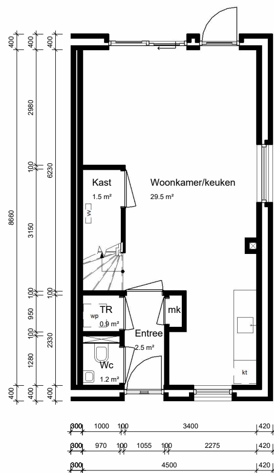
begane grond
