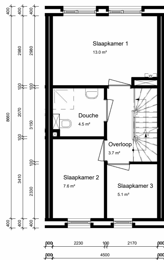
eerste verdieping
