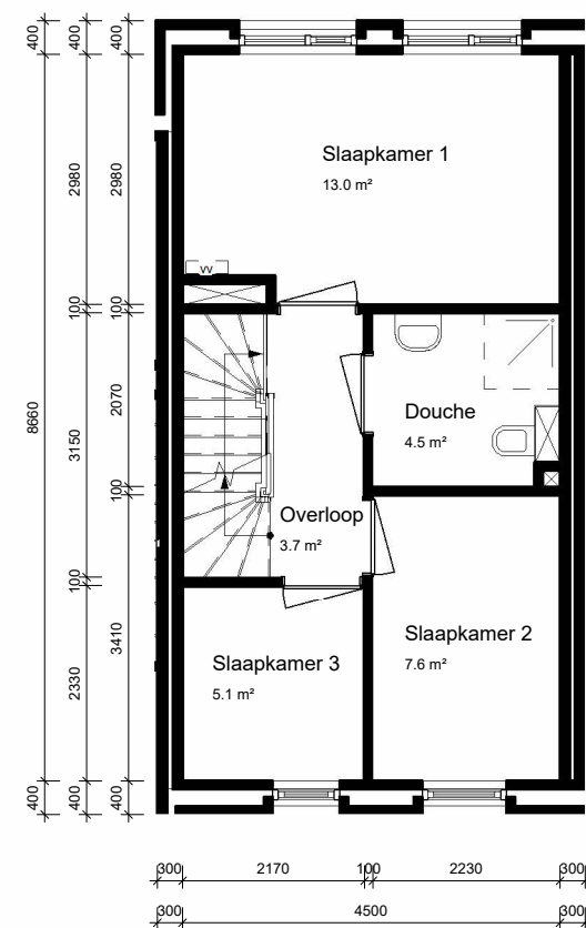
eerste verdieping
