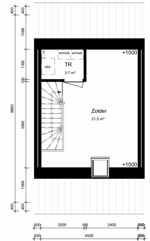
tweede verdieping
