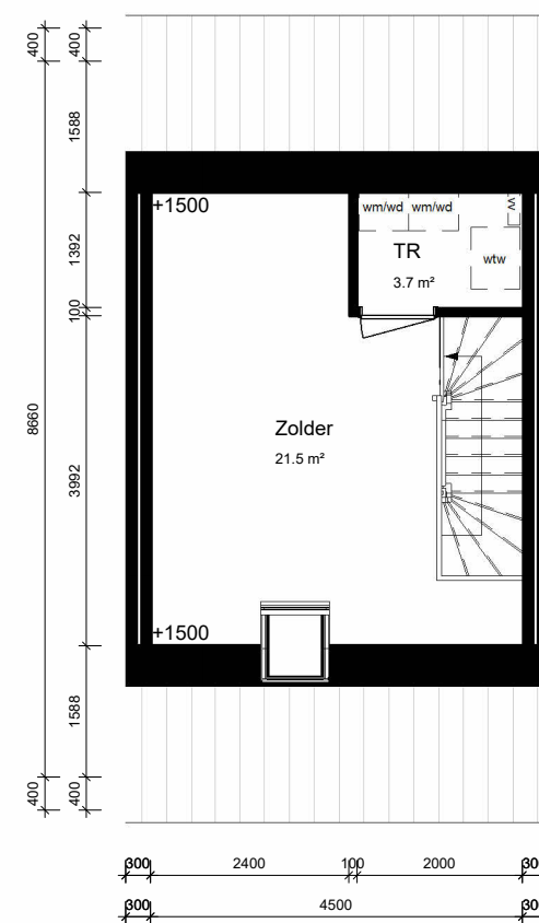
tweede verdieping
