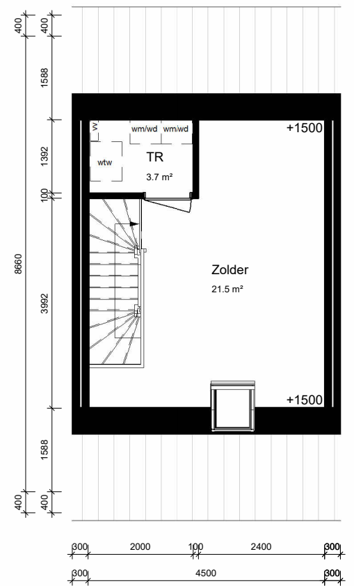
tweede verdieping
