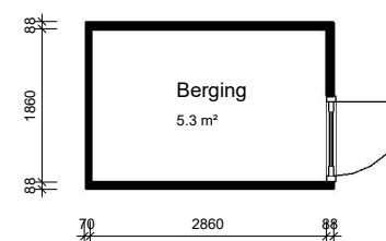
begane grond
