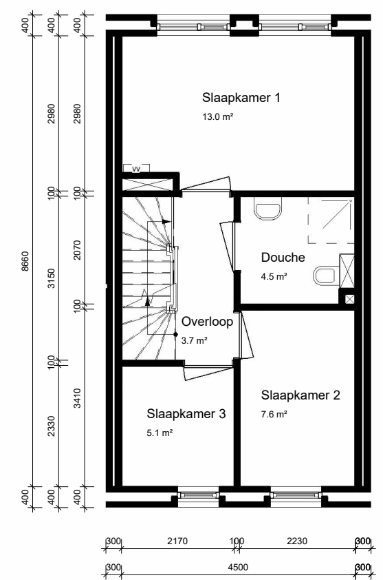
eerste verdieping
