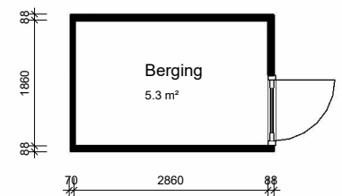
begane grond
