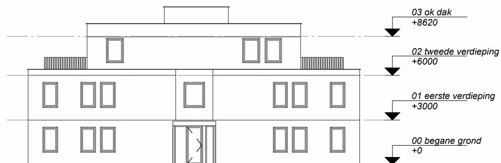
zuidgevel
