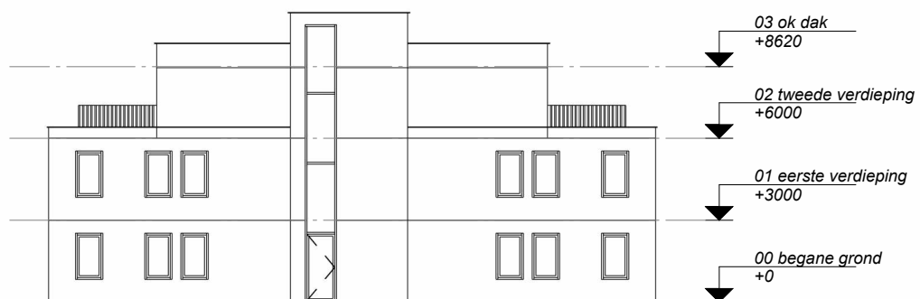
noordgevel
